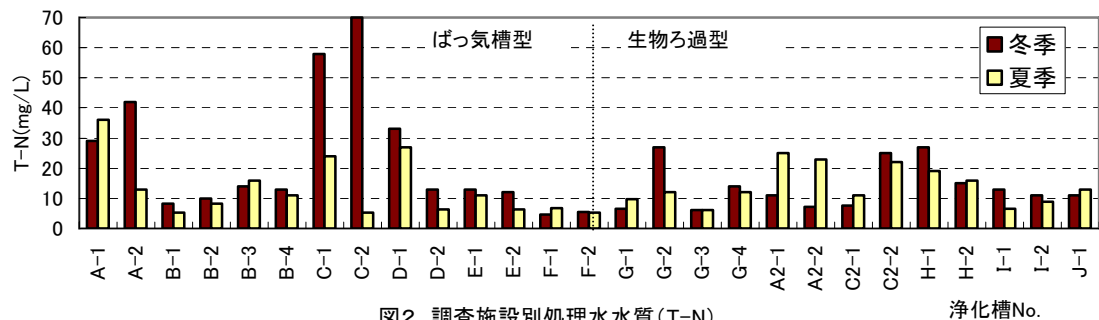
図2 調査施設別処理水水質(T-N)
