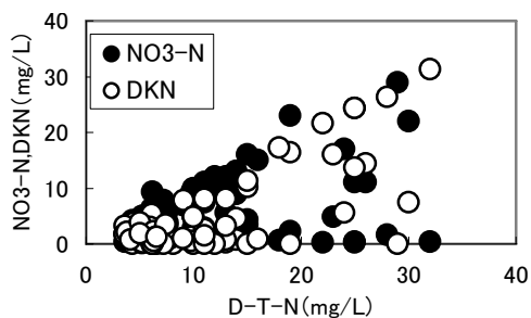
図3 処理水D-T-NとNO3-N,DKNの関係
