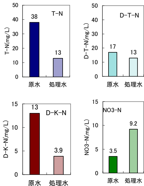
図4 嫌気ろ床槽(原水)と沈殿槽(処理水)の水質(N=28)
