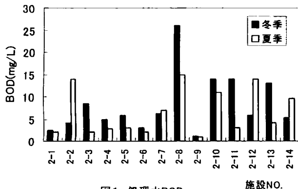
図1 処理水BOD
