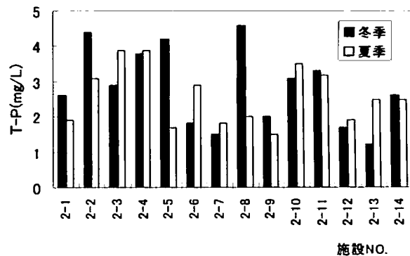
図4 処理水T-P
