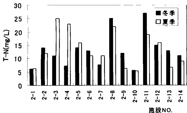
図3 処理水T-N
