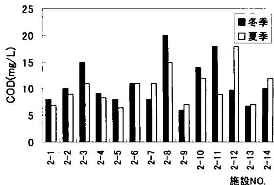
図2 処理水COD
