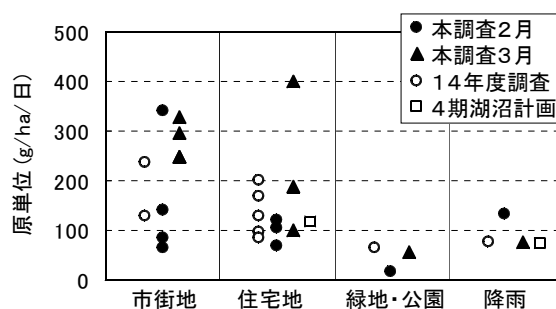
図1 COD原単位
