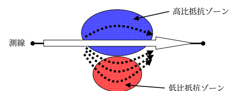
図7 隣接する低比抵抗ゾーンからの影響
