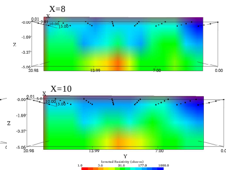
図6 2D 探査測線の周辺の 3D 探査による断面 X=8 断面 (上)、X=10 断面 (下)
