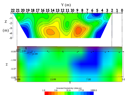
図3 比抵抗断面図 Y-Z 断面(X=3) 2D 探査 (上) 3D 探査 (下)
