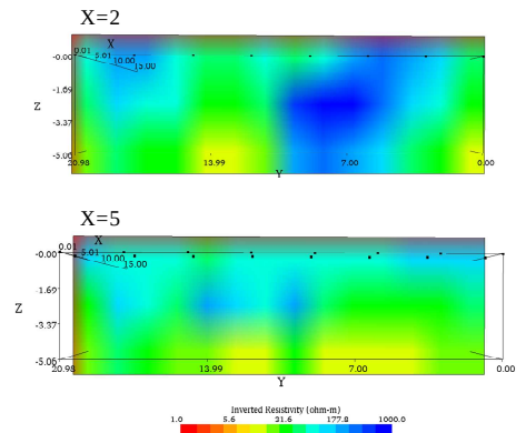
図4 2D 探査測線の周辺の 3D 探査による断面 X=2 断面 (上)、X=5 断面 (下)
