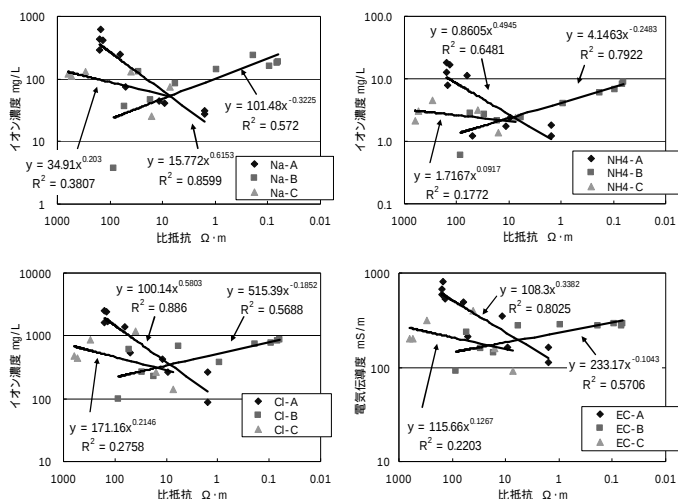
図5 比抵抗と溶出濃度の比較
