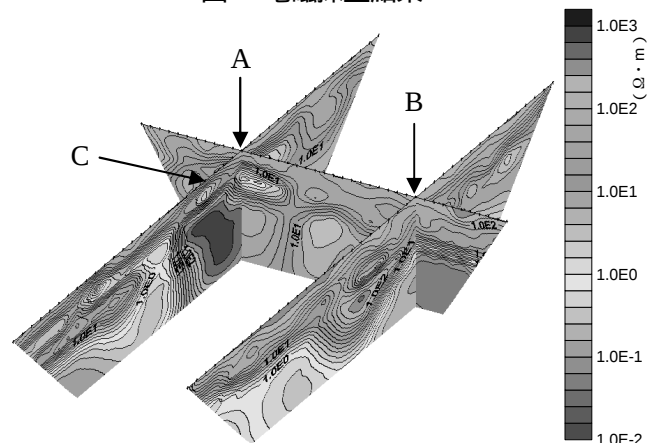
図2 電気探査結果
