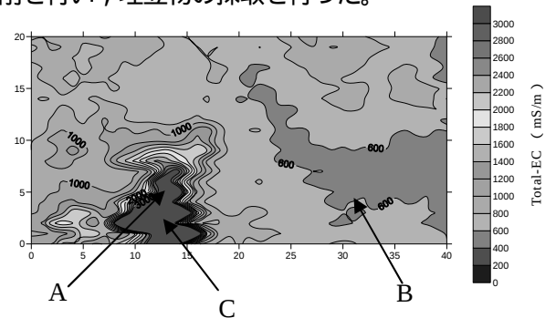
図1 電磁探査結果
