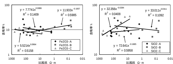
図4 比抵抗と含有量の比較
