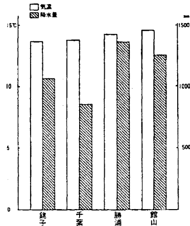
平均気温と降水量(59年)
