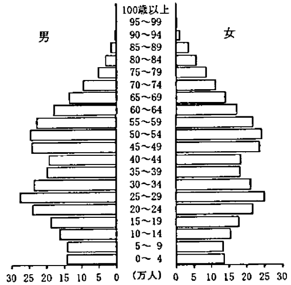
人口構造 (11. 4. 1)
