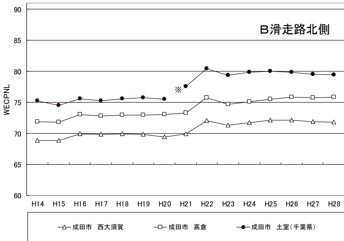
図 11 B滑走路周辺 年間WECPNLの経年変化
