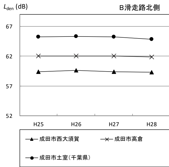
図9 B滑走路周辺年間 L_{den} 値経年変化
