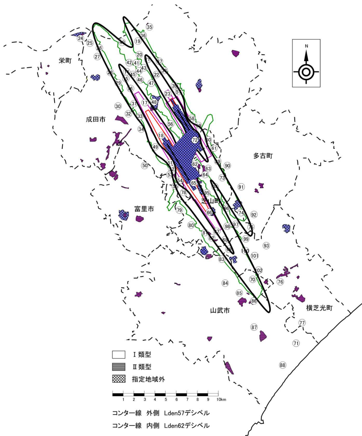
図5 年間 L_{den} 値コンター図
