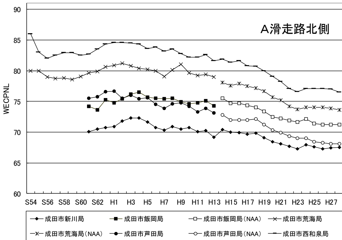
図 10 A 滑走路周辺 年間WECPNLの経年変化
