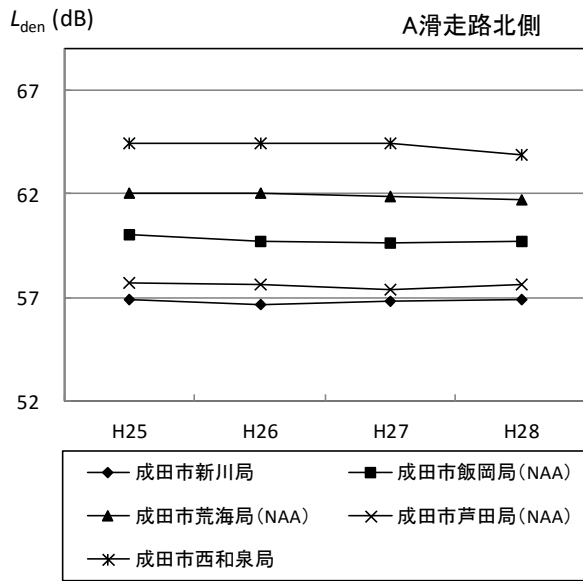
図8 A滑走路周辺年間 L_{den} 値経年変化
