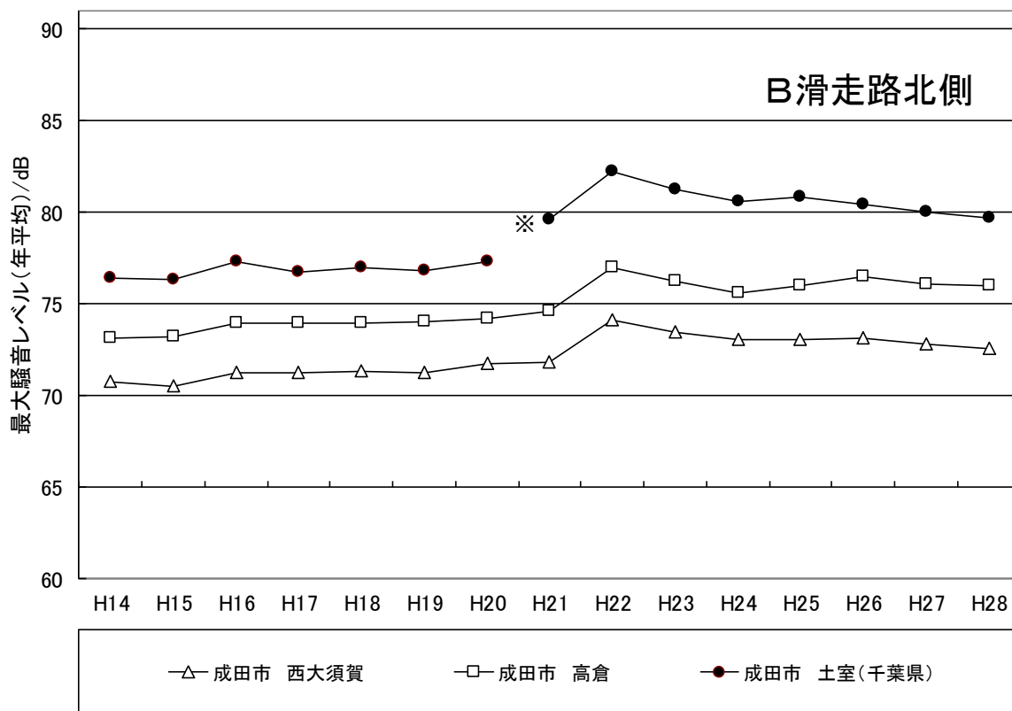
図7 B滑走路周辺 最大騒音レベル（年平均値）の経年変化
