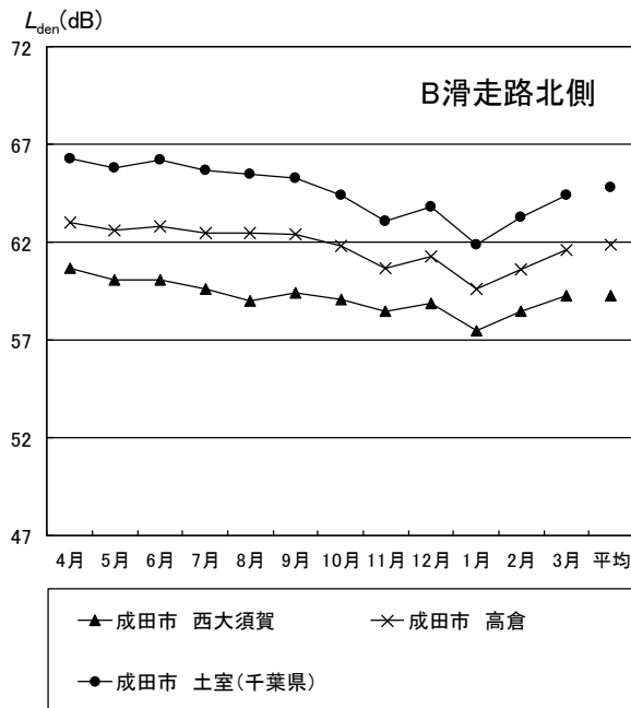
図4 B滑走路周辺 月間 L_{den} 値
