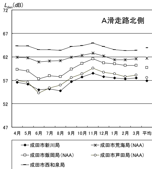
図3 A滑走路周辺 月間 L_{den} 値
