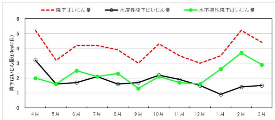
図3-2 降下ばいじん量、水溶性降下ばいじん量、水不溶性降下ばいじん量の経月変化
