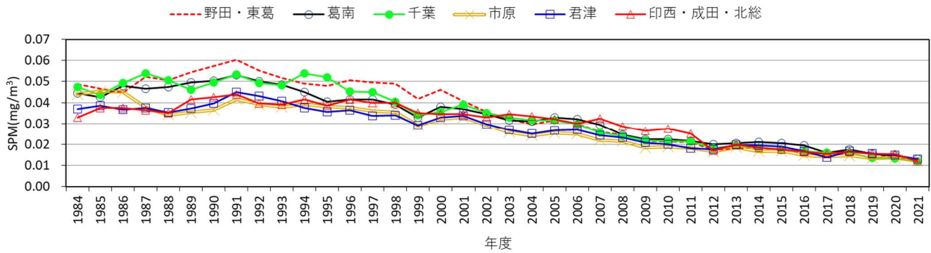
図2-6-7 SPM年平均値の推移(一般局)
