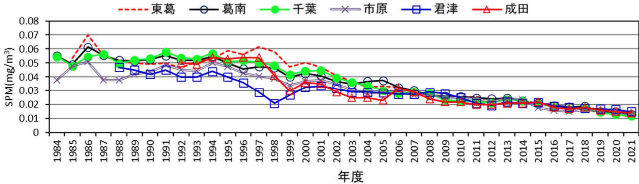
図2-6-8 SPM年平均値の推移(自排局)
