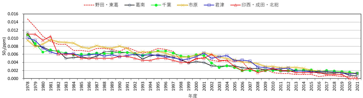
図2-1-5 SO 2 年平均値の推移(一般局)
