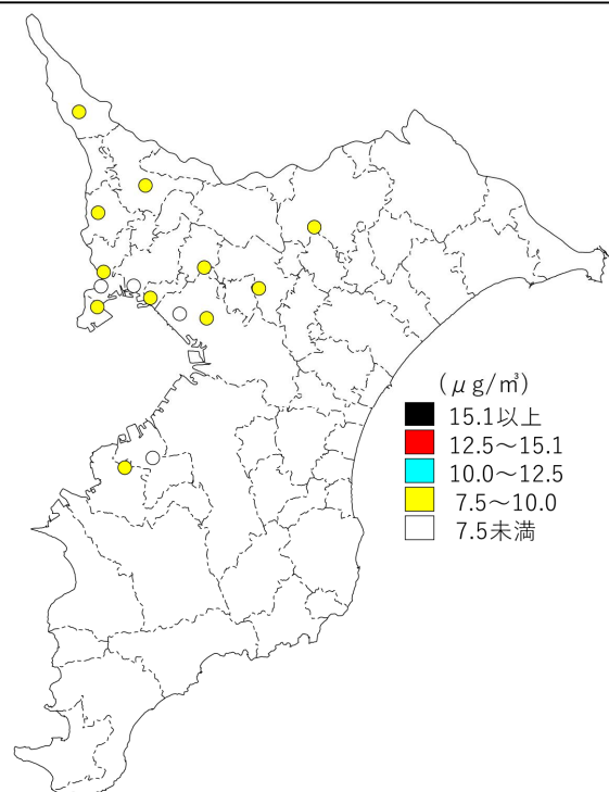
図2-7-2 PM2.5年平均値分布(自排局)
