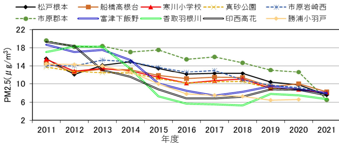
図2-7-5 PM2.5年平均値の推移(一般局)
