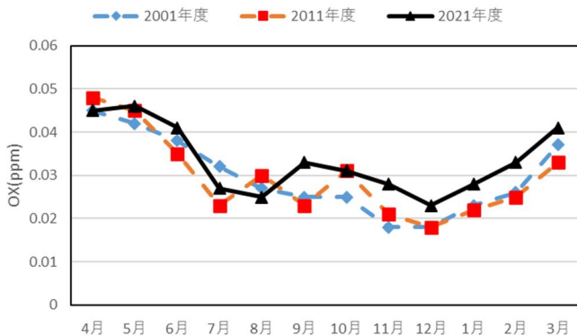
図 2-5-3 Ox月平均値の経月変化
