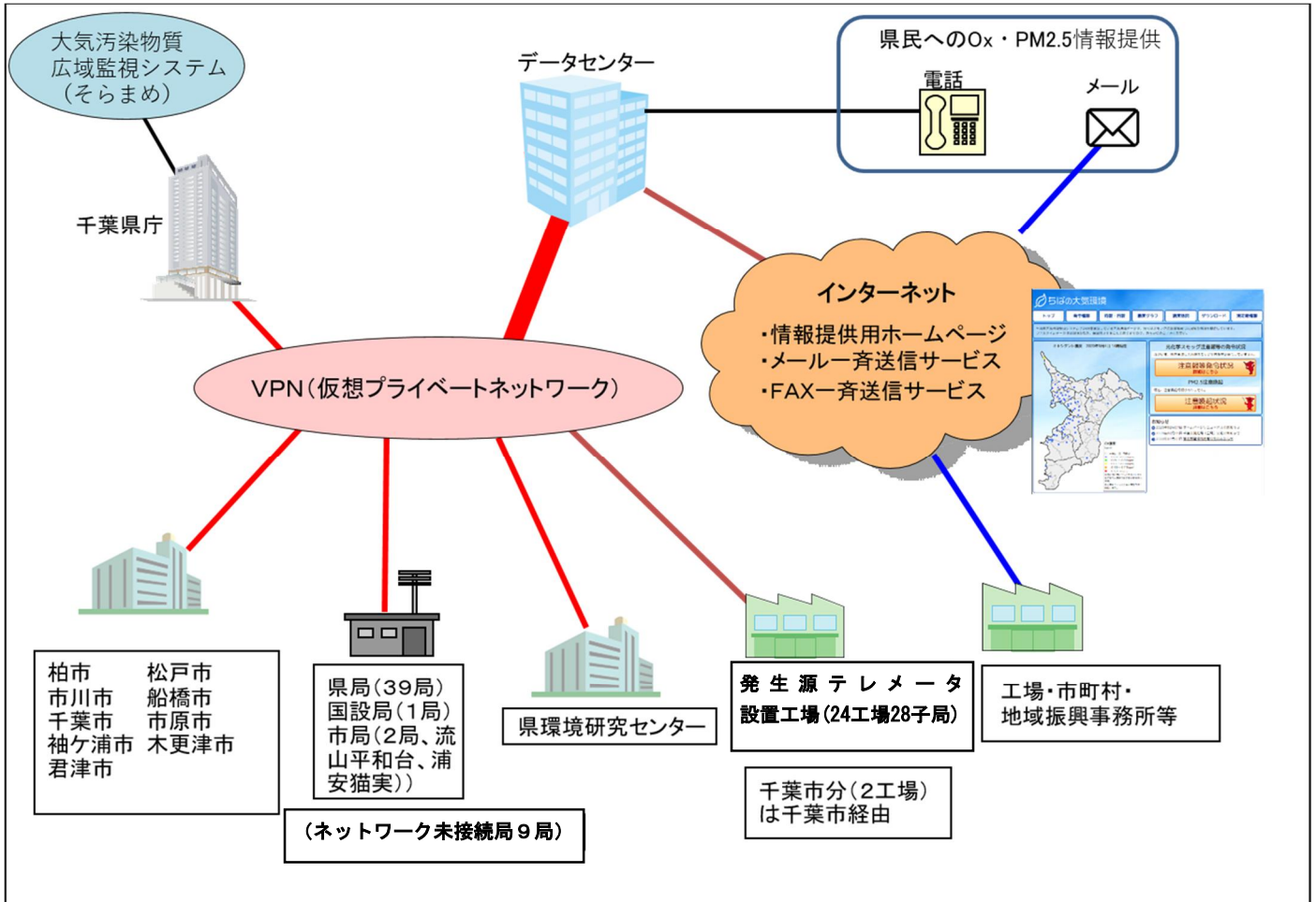
千葉県大気情報管理システム ネットワーク構成図(2021年4月1日現在)
