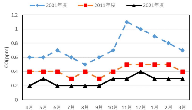
図2-4-4 CO月平均値の経月変化(自排局)
