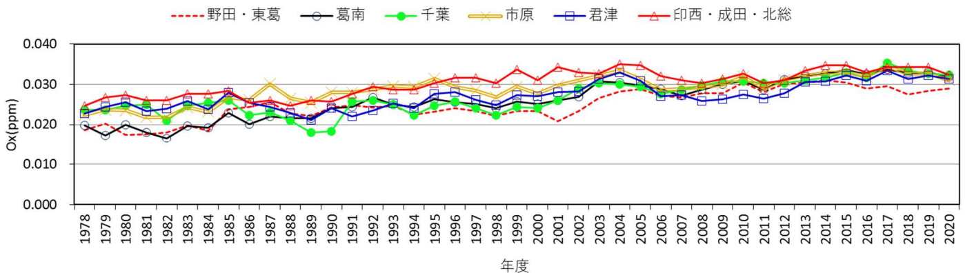
図 2-5-5 Ox年平均値の推移
