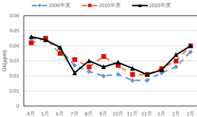
図 2-5-3 Ox月平均値の経月変化
