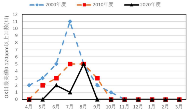
図 2-5-4 Ox日最高値0.120ppm以上日数の推移
