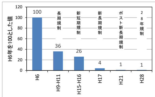
図2-11 ディーゼル重量車(3.5トン超)規制強化の推移(PM)
