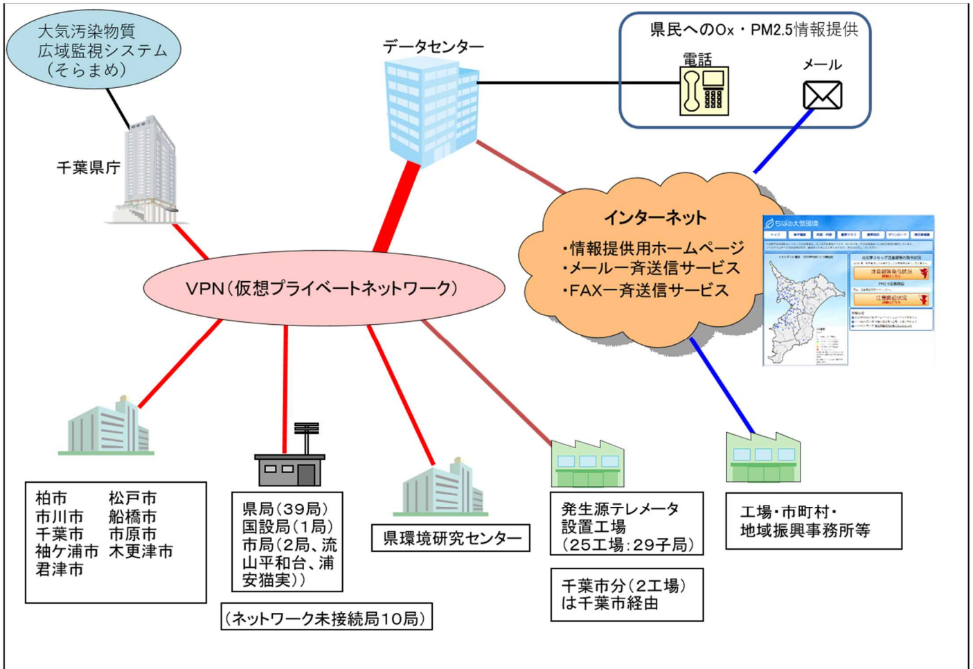
千葉県大気情報管理システム ネットワーク構成図(2020年4月1日現在)
