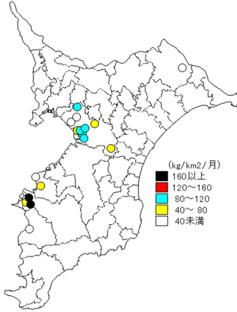
図3-7 Al量の分布
