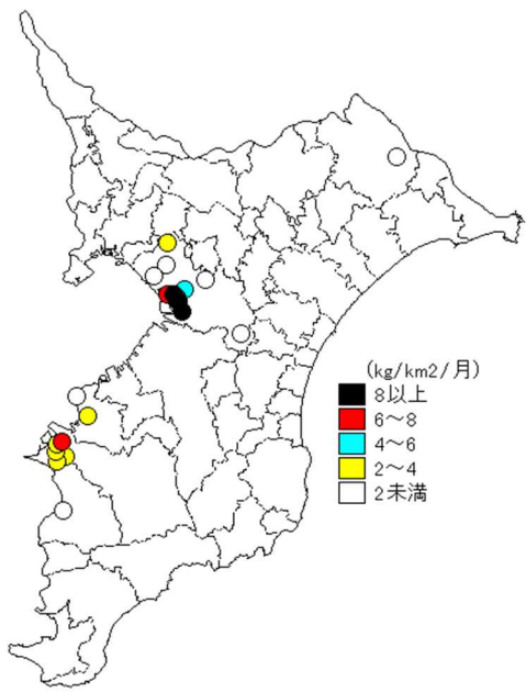
図3-9 Mn量の分布
