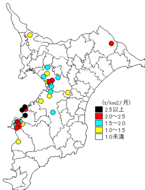
図3-5 水溶性降水ばいじん量の分布
