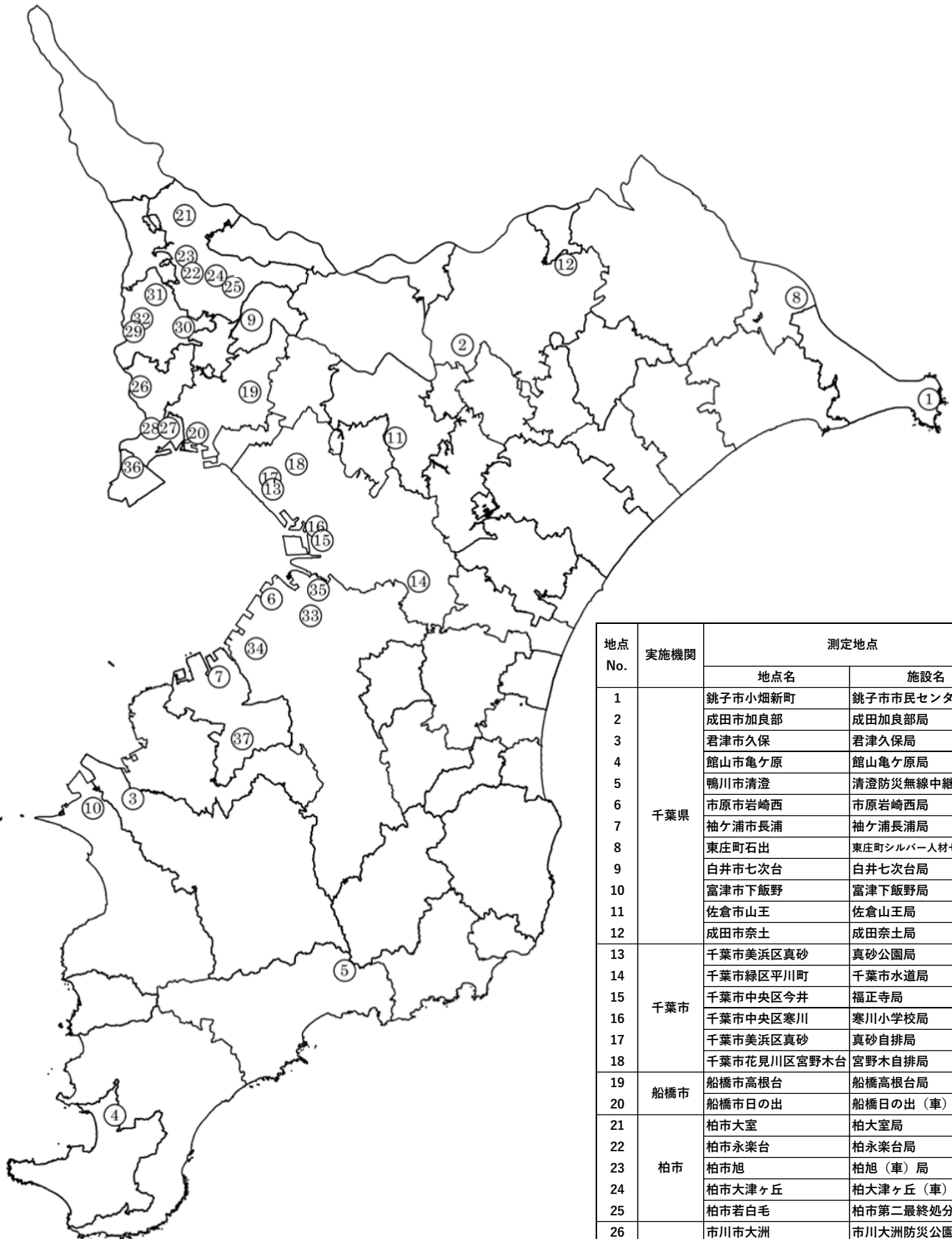
図2 有害大気汚染物質等測定地点図
