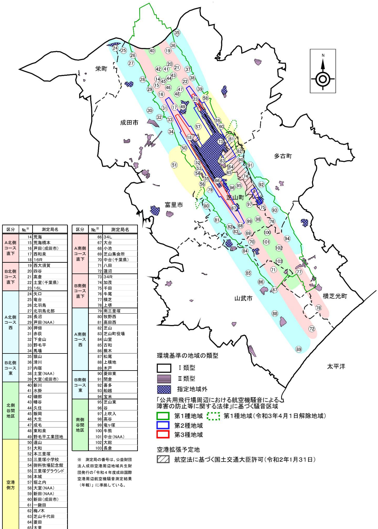
図1 成田空港周辺における航空機騒音の固定測定局
