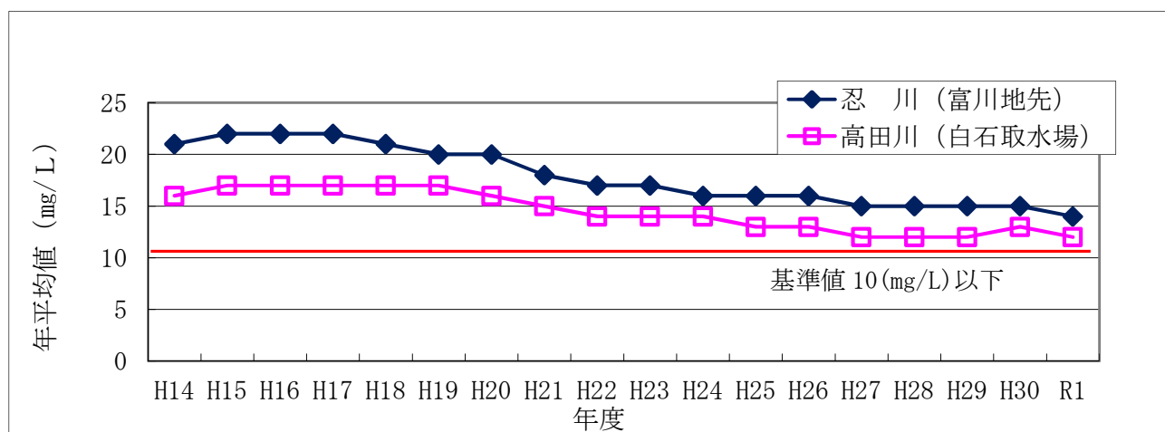
図 1 忍川及び高田川の硝酸性窒素及び亜硝酸性窒素の経年変化
