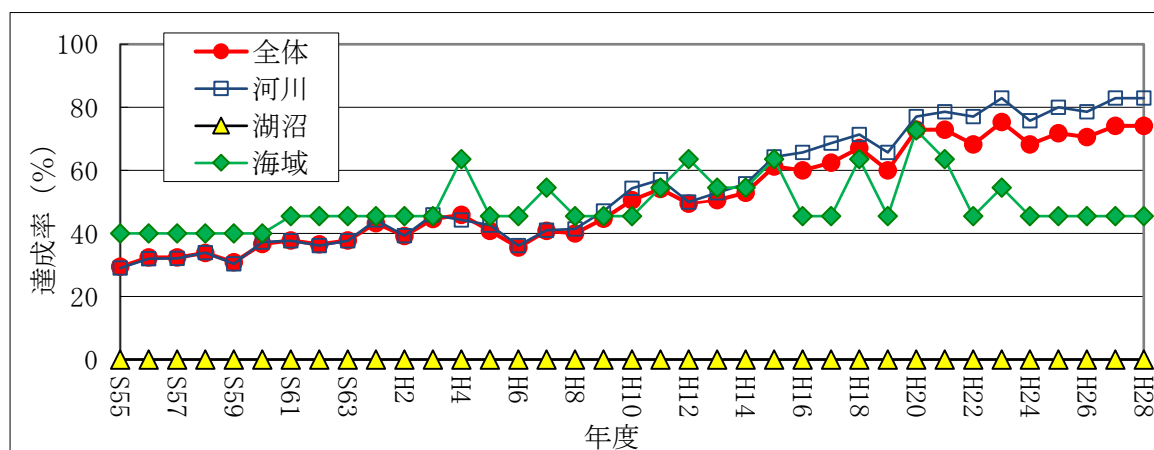
図2 環境基準達成率の推移 (BOD・COD)
