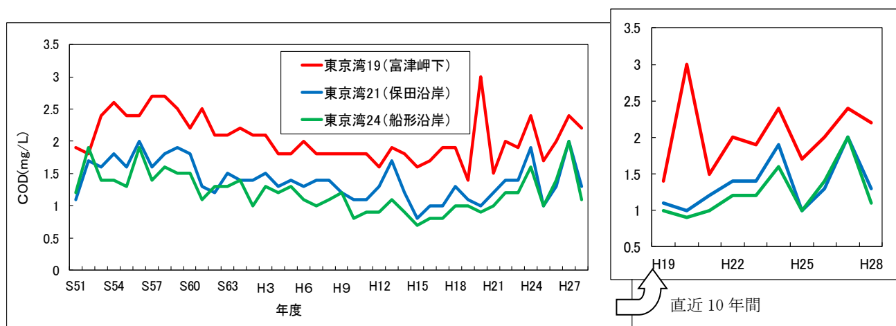
図 3-7 東京湾内房の水質経年変化 (COD 年平均值)
