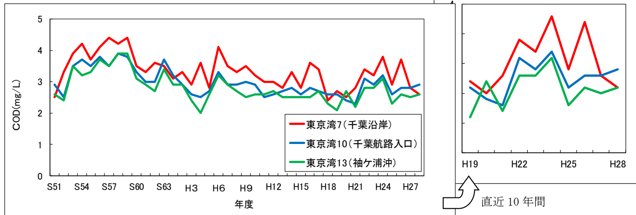
図 3-6 東京湾内湾の水質経年変化 (COD 年平均值)
