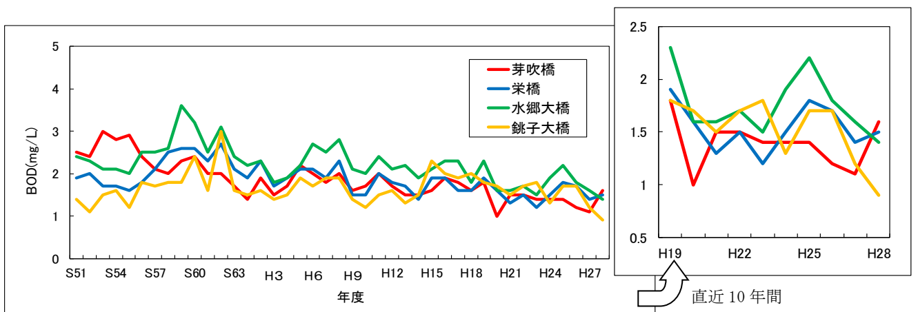
図3-2 利根川の主要地点の水質経年変化（BOD年平均値）
