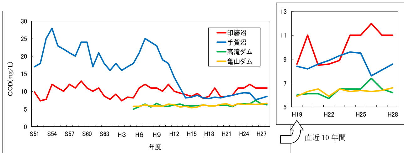
図 3-5 県内湖沼の水質経年変化 (COD年平均值)
