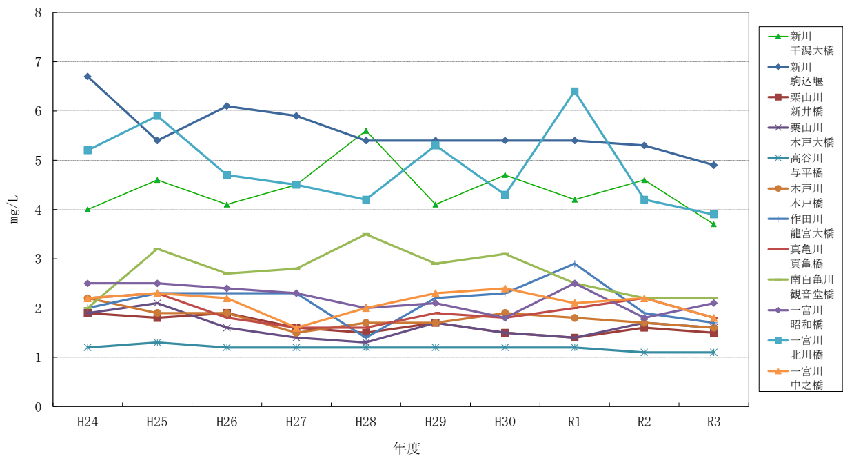
図1-12 九十九里海域流入河川（環境基準点）水質（BOD年平均値）経年変化
