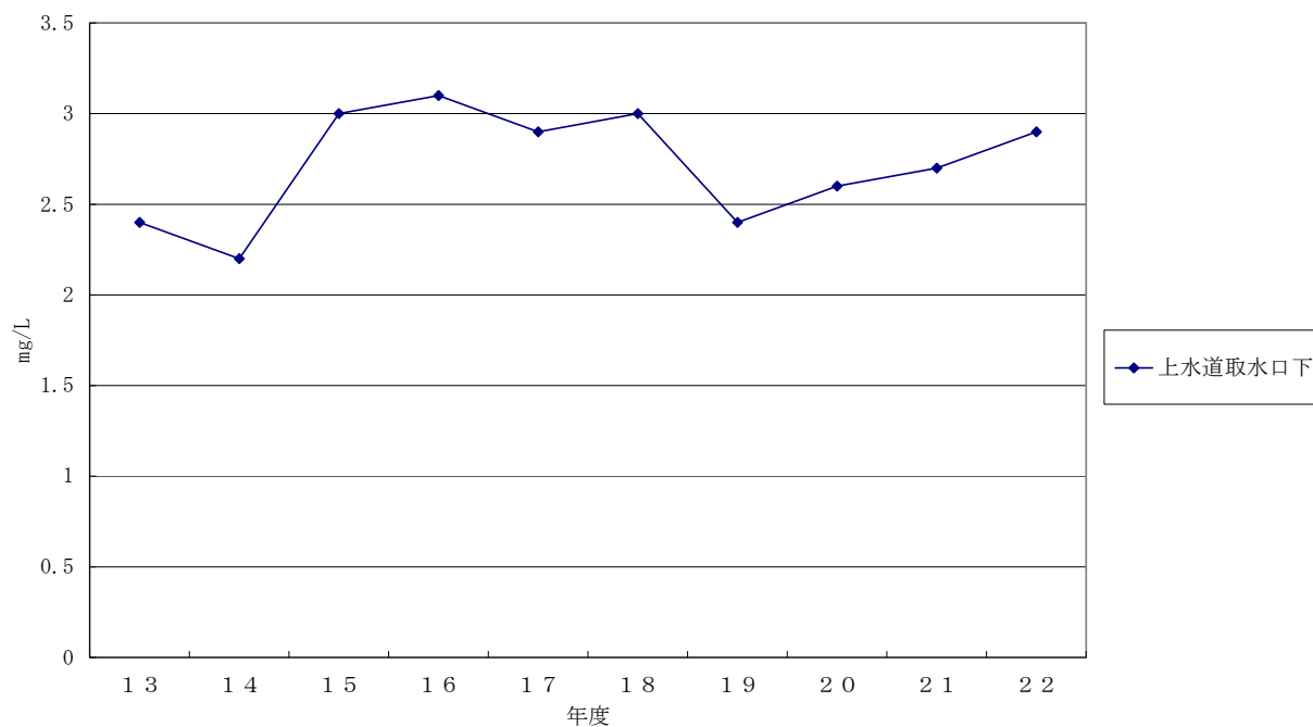
図1-18 全窒素推移
