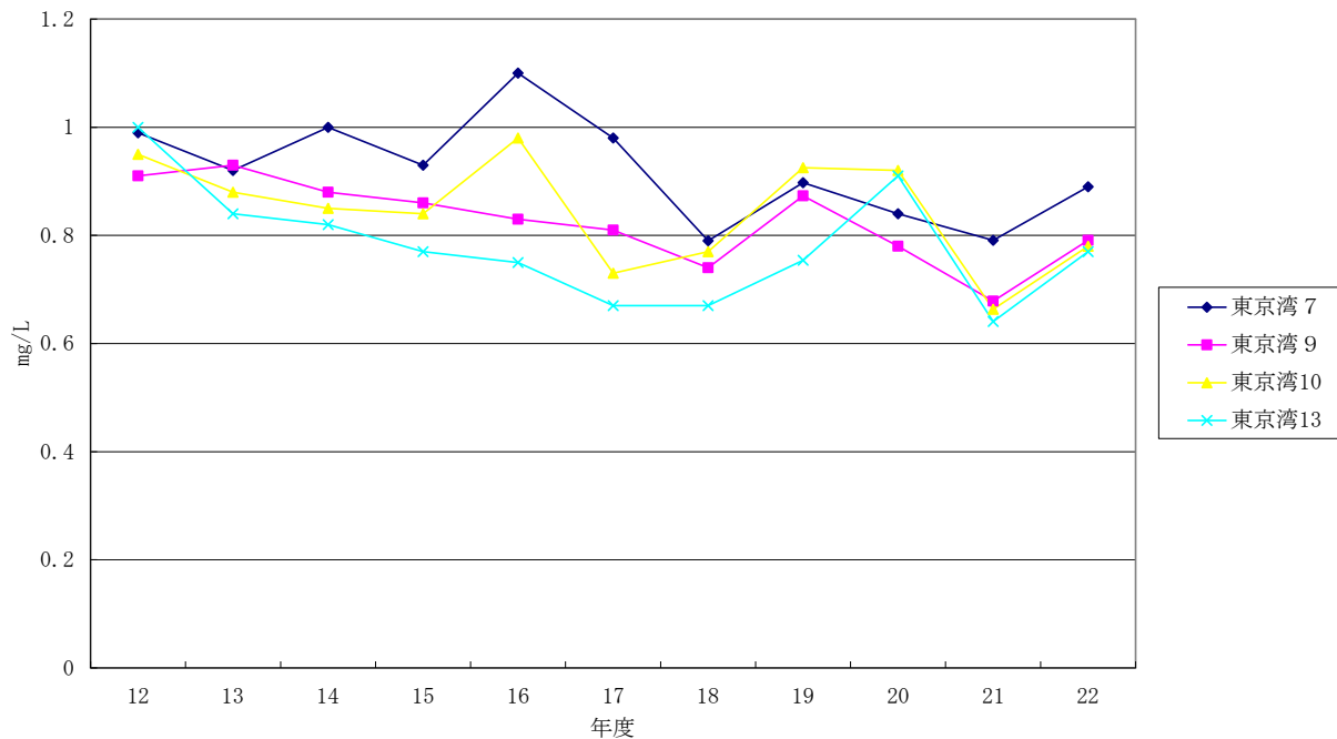
図1-26 全窒素推移
