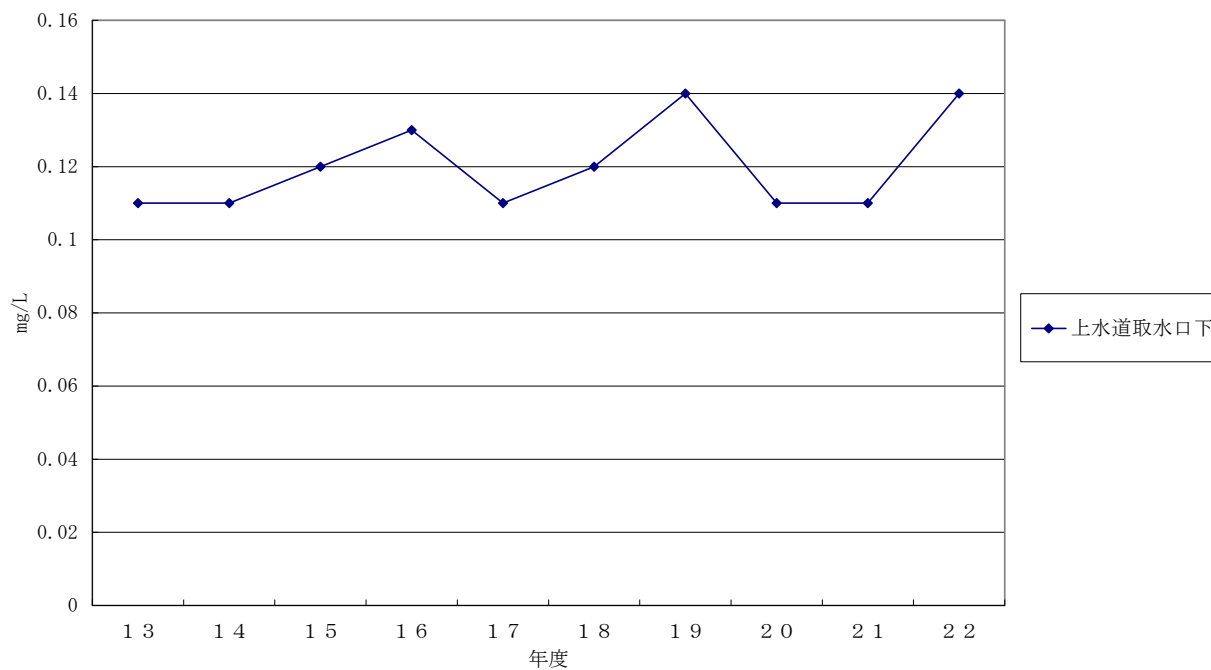
図1-19 全りん推移
