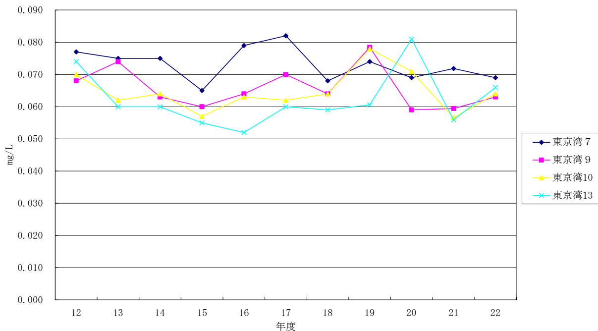
図1-27 全りん推移
