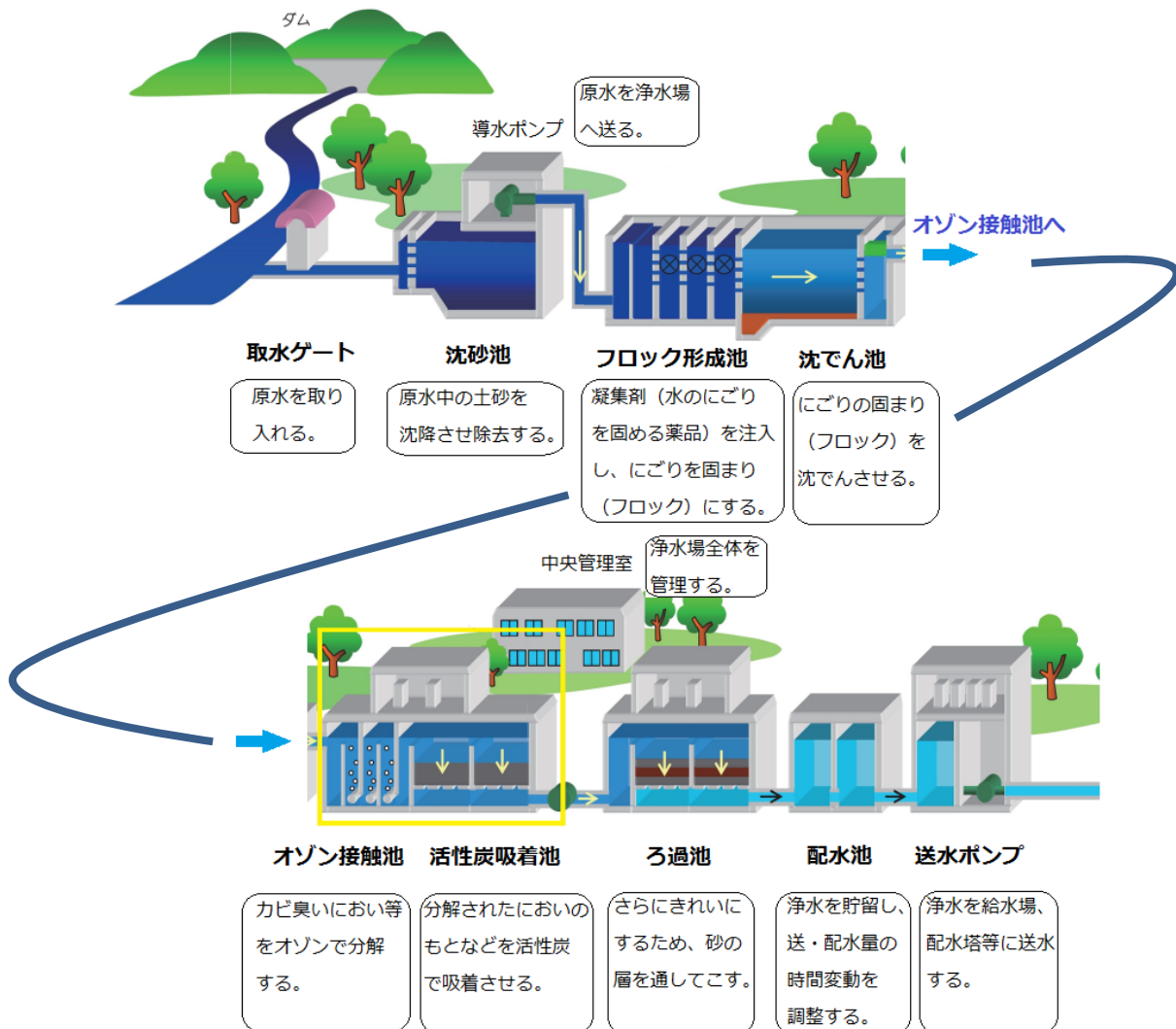
図3-8 浄水処理の概要（黄色の枠内が高度浄水処理）
