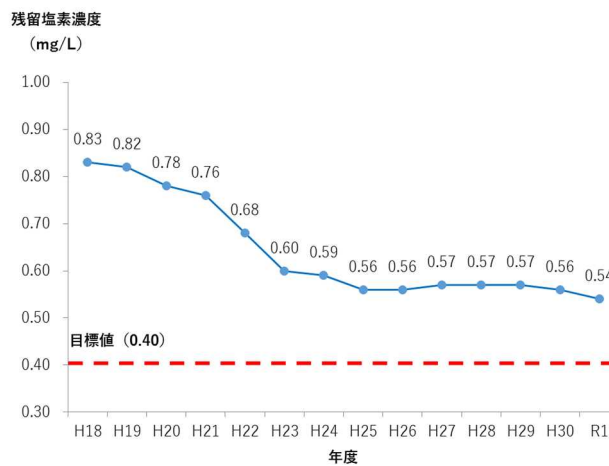
図〇—〇 給水区域内の残留塩素濃度の推移
