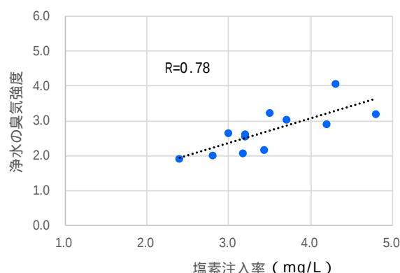
図 1-8 臭気強度と塩素注入率の関係の例
