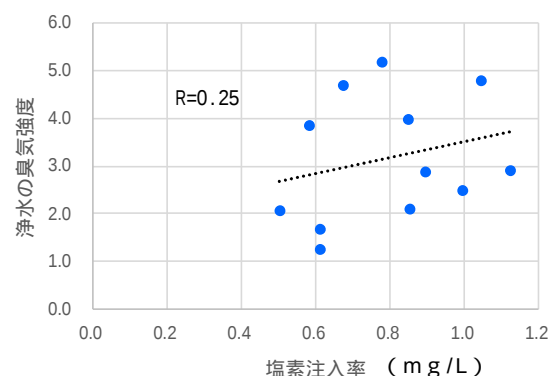
浄水の臭気強度と中 + 後塩素注入率の関係 ( ちば野菊の里浄水場 )
