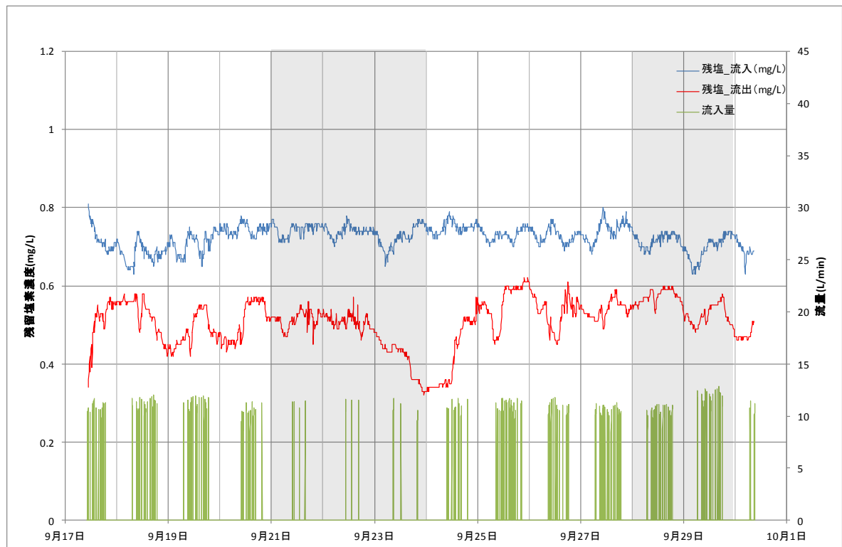
図 1.1.1 残留塩素濃度・流量 (No. 2_夏期)
