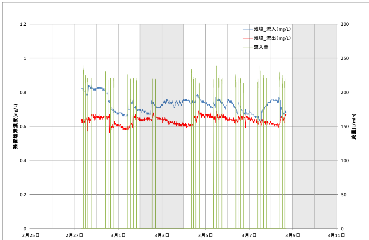
図 1.3.3 残留塩素濃度・流量 (No. 8_冬期)
