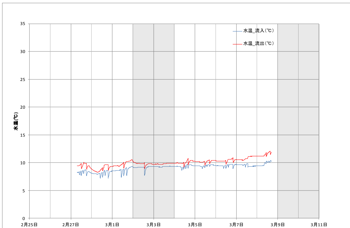
図 1.3.4 水温 (No. 8_冬期)
