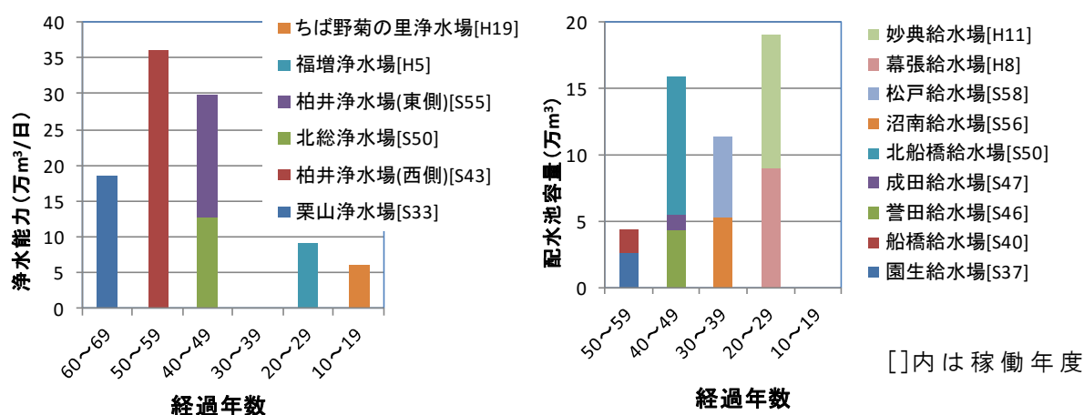
図 4 浄水能力及び配水池容量の整備状況
