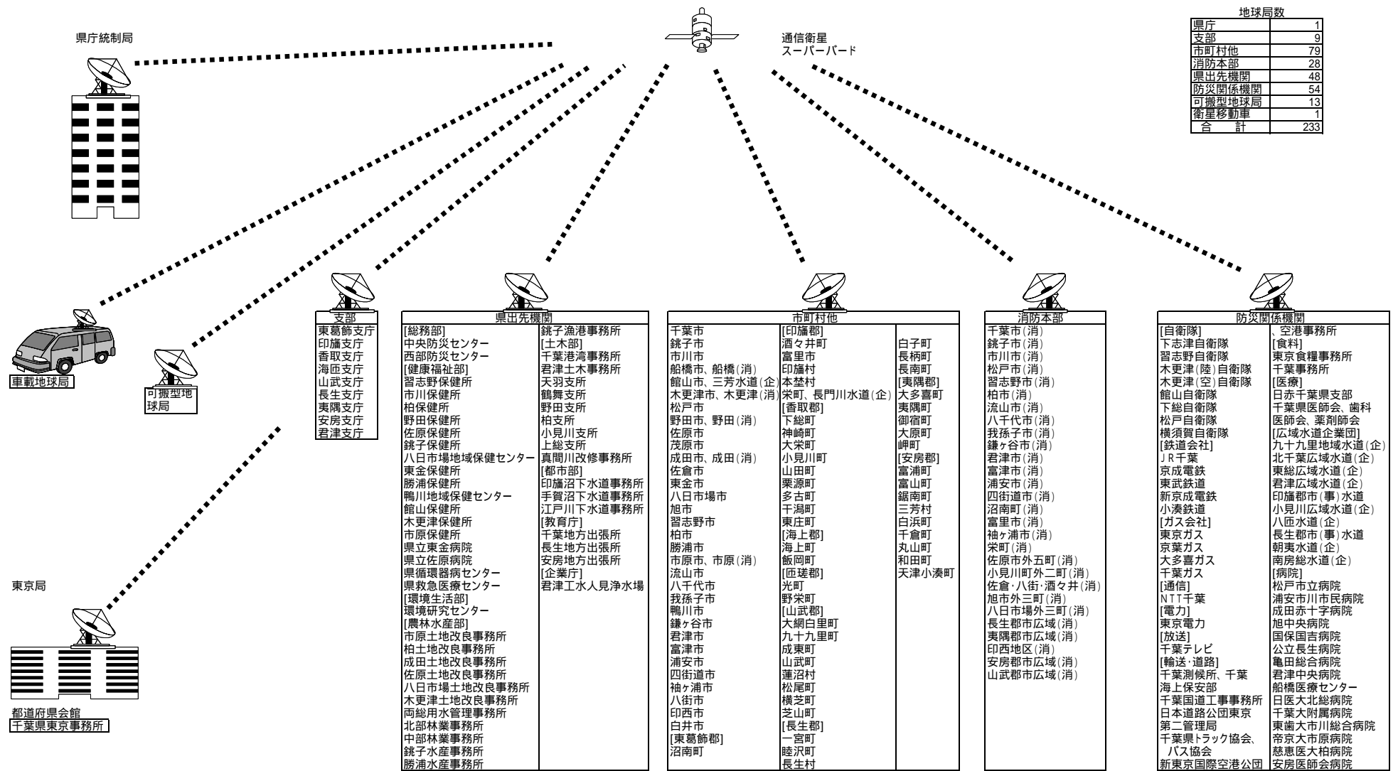
図2 防災行政無線衛星系回線構成図(平成15年4月現在)
