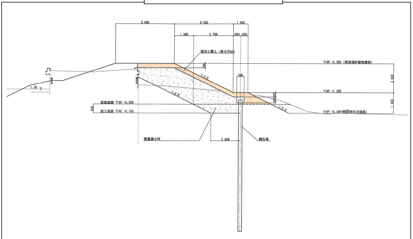
a - a' 断面図 (参考図)
