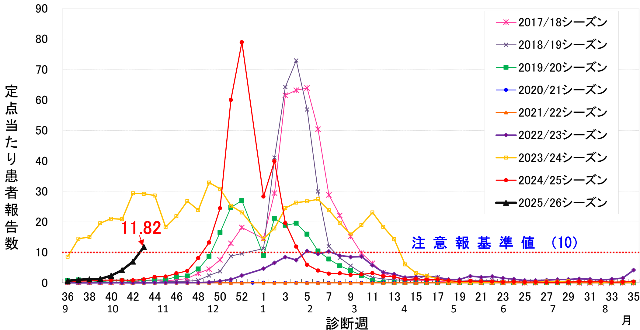
2017/18シーズンから2025/26シーズン（2025年第43週）までのインフルエンザ定点当たり患者報告数の推移
