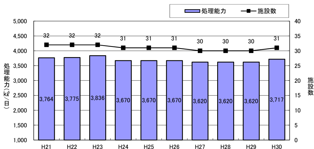
図-16 し尿処理施設の推移
