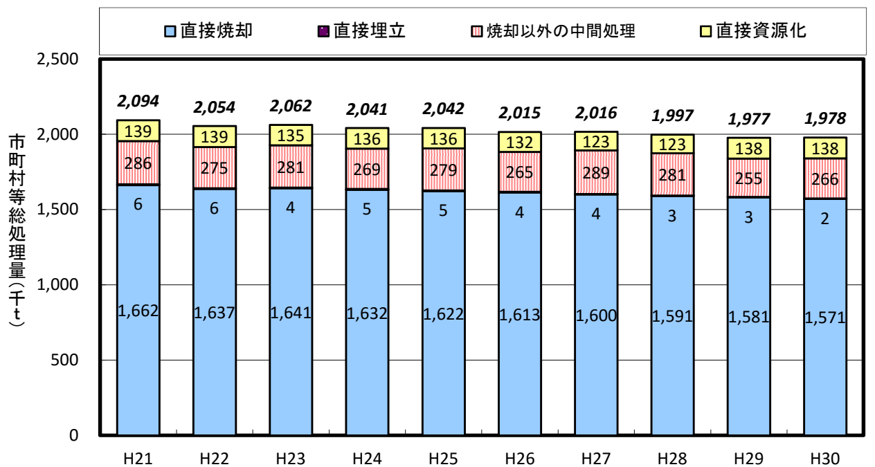
図-4 ごみ処理方法の推移
