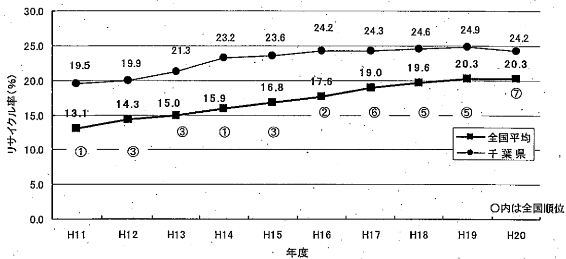
図－９ リサイクル率の推移
