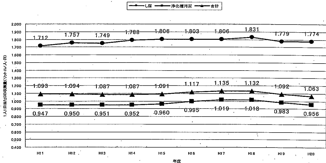
図一15 し尿及び浄化槽汚泥の1人1日あたりの収集量の推移
