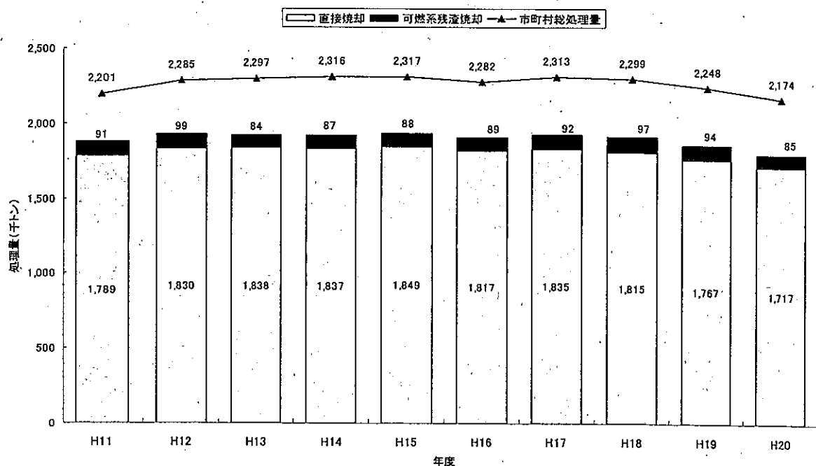
図一5 焼却処理総量の推移
