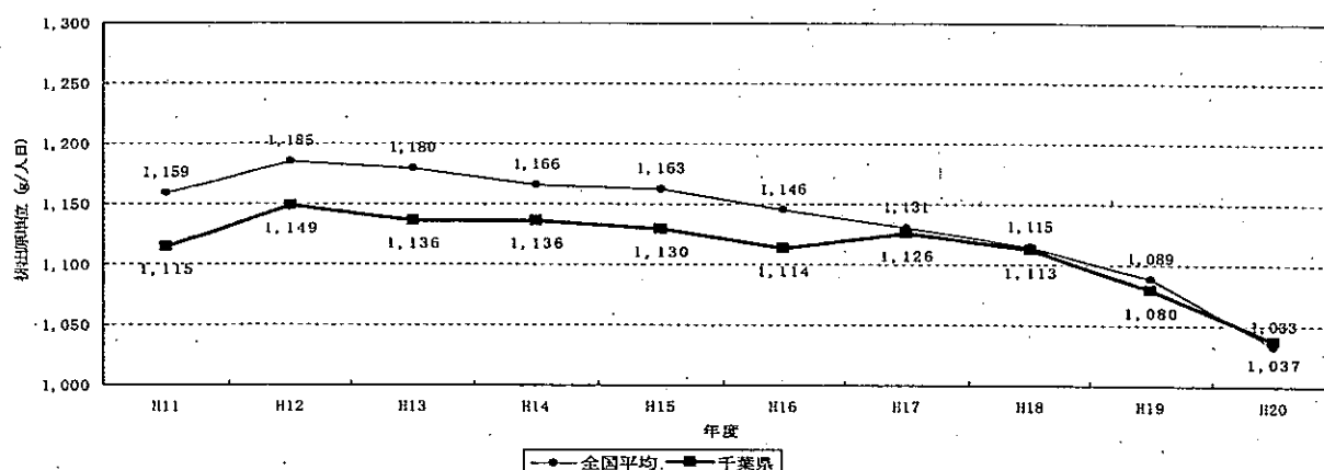
図-2 1人1日当たりのごみの排出量全国との比較
