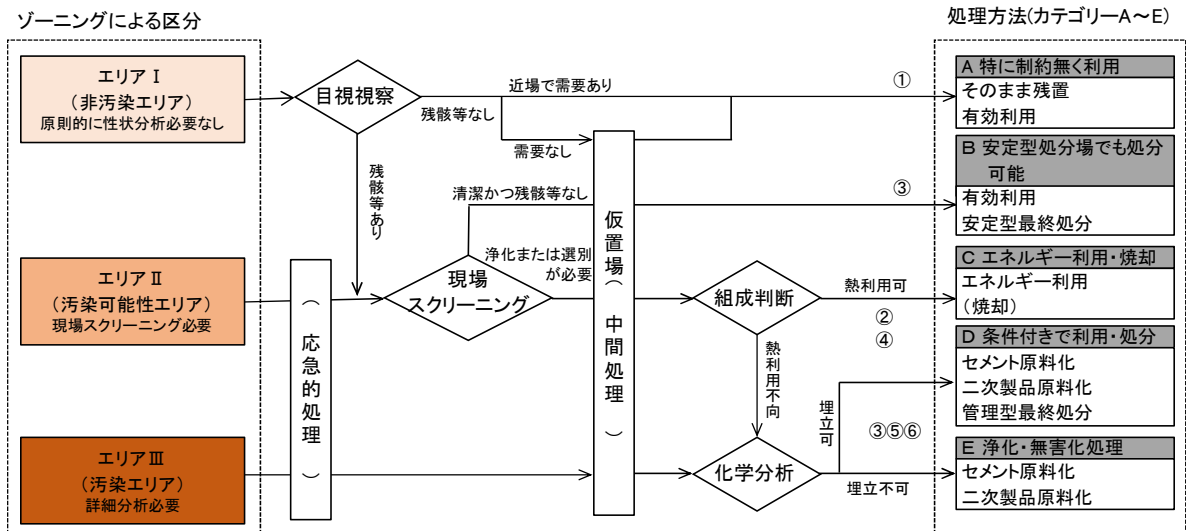
図表 2-24 津波堆積物の処理フロー（全体）
