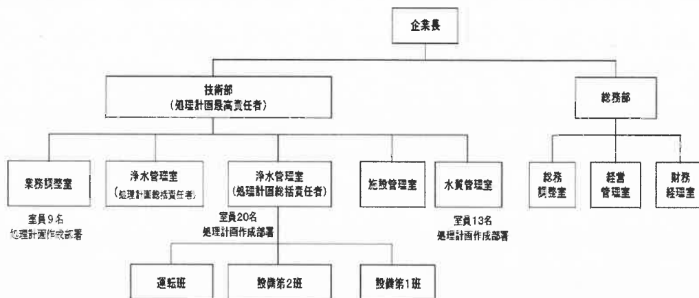
(管理体制図)
