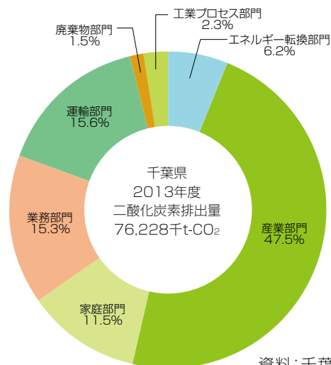
千葉県の二酸化炭素排出量の部門別構成比
