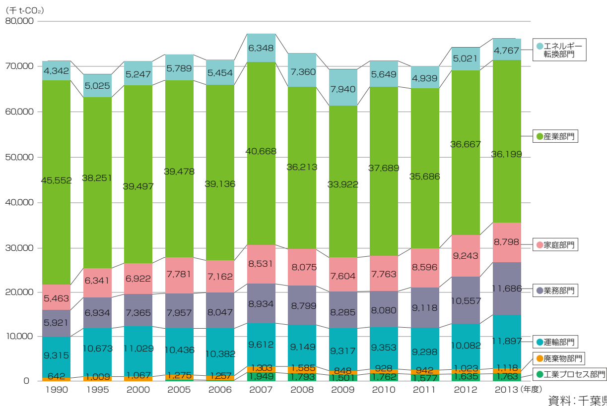
千葉県における部門別二酸化炭素排出量の推移
