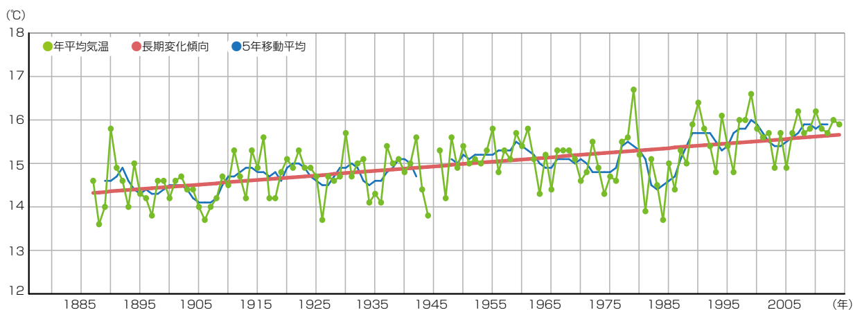
銚子地方気象台における年平均気温の長期変化
