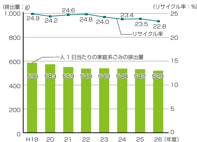
県民一人1日当たりの家庭系ごみの排出量と 県内の一般廃棄物のリサイクル率の推移
