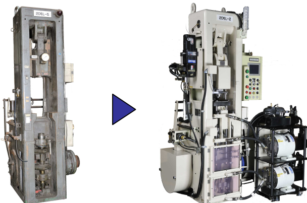
粉末サーボプレス改造事例
