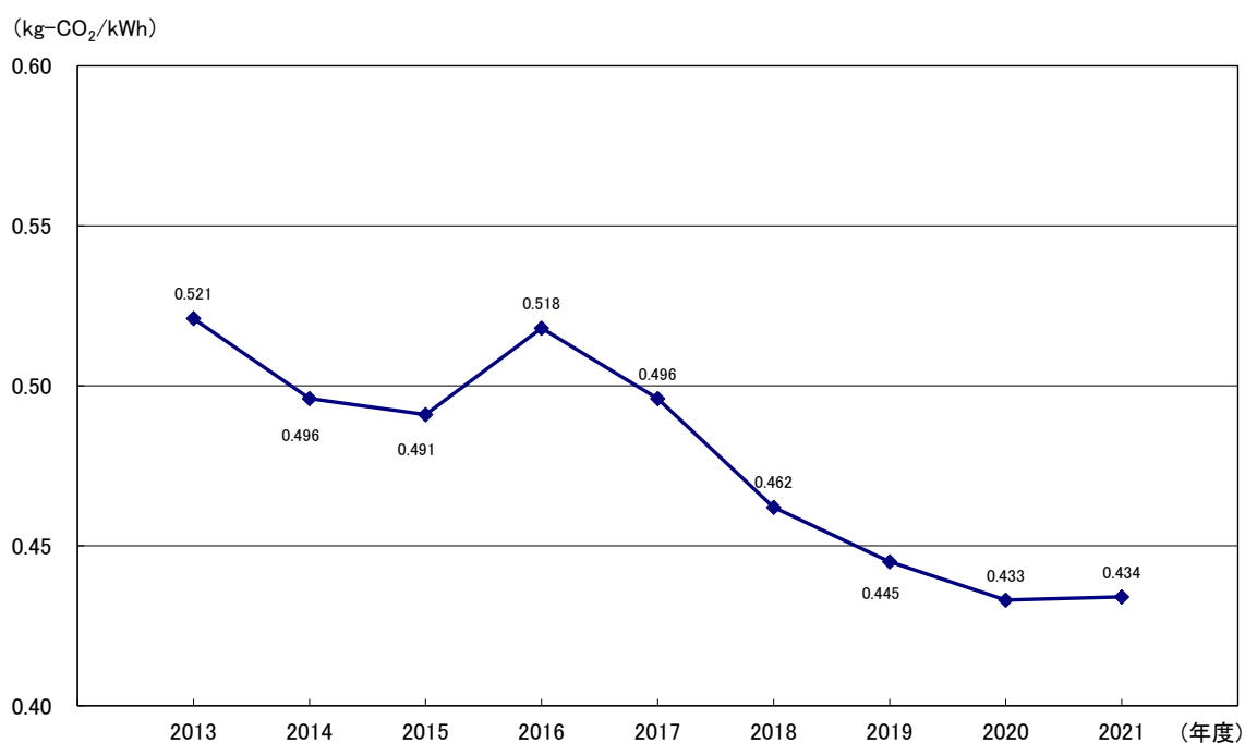
図 6 東京電力パワーグリッド株式会社の電力排出係数（調整後）推移
