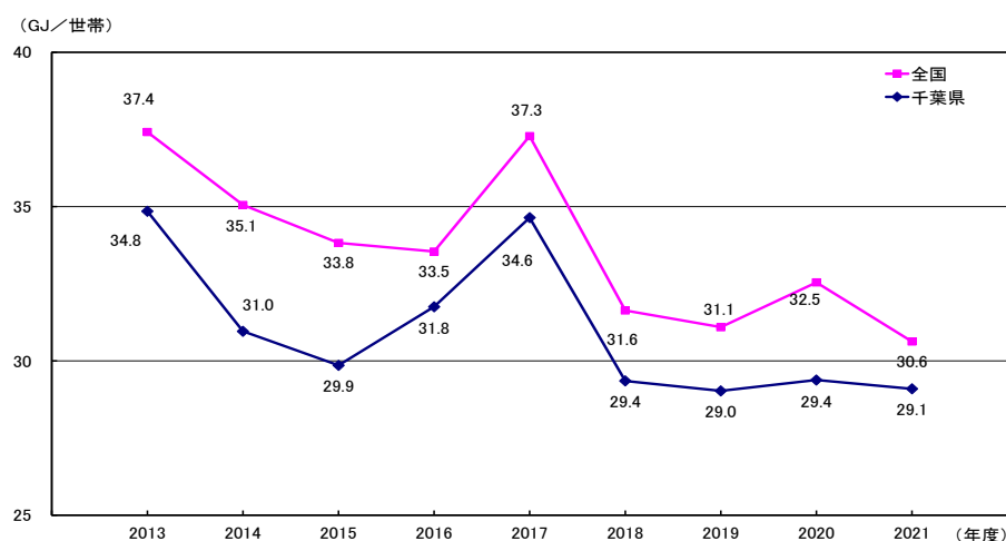
図 5-1 世帯当たりエネルギー消費量の推移
