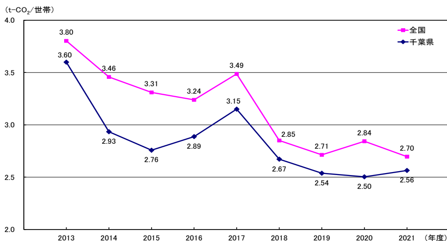
図 5-2 世帯当たり二酸化炭素排出量の推移
