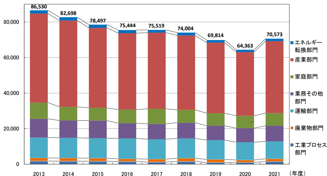
図3 千葉県における二酸化炭素排出量の推移
