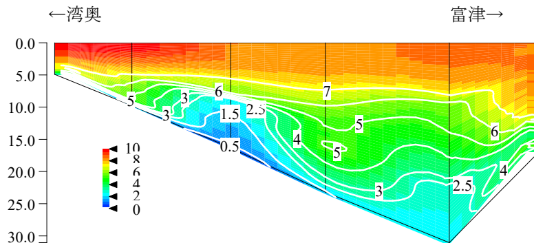
図2 縦断ラインでのDO鉛直分布
