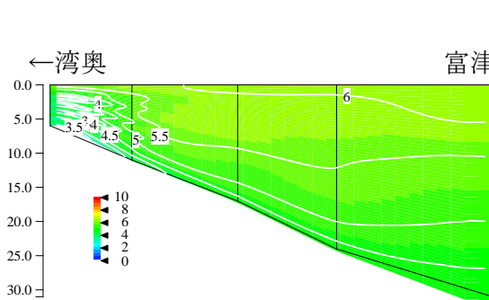
図2 縦断ラインでのDO鉛直分布
