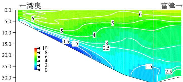
図2 縦断ラインでのDO鉛直分布
