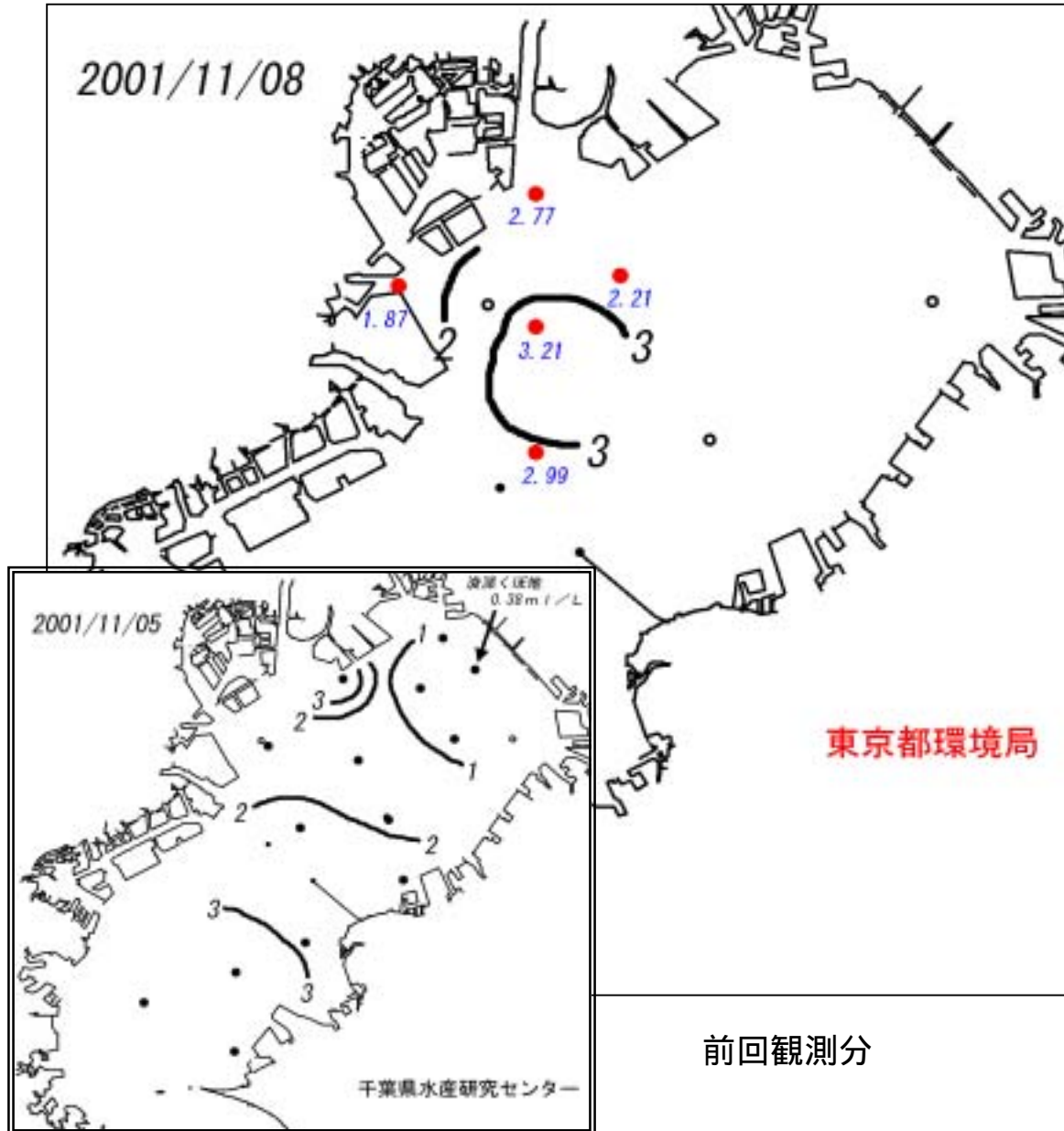
図 底層の溶存酸素量分布 (ml / L:速報値) 平成13年11月8日観測分
