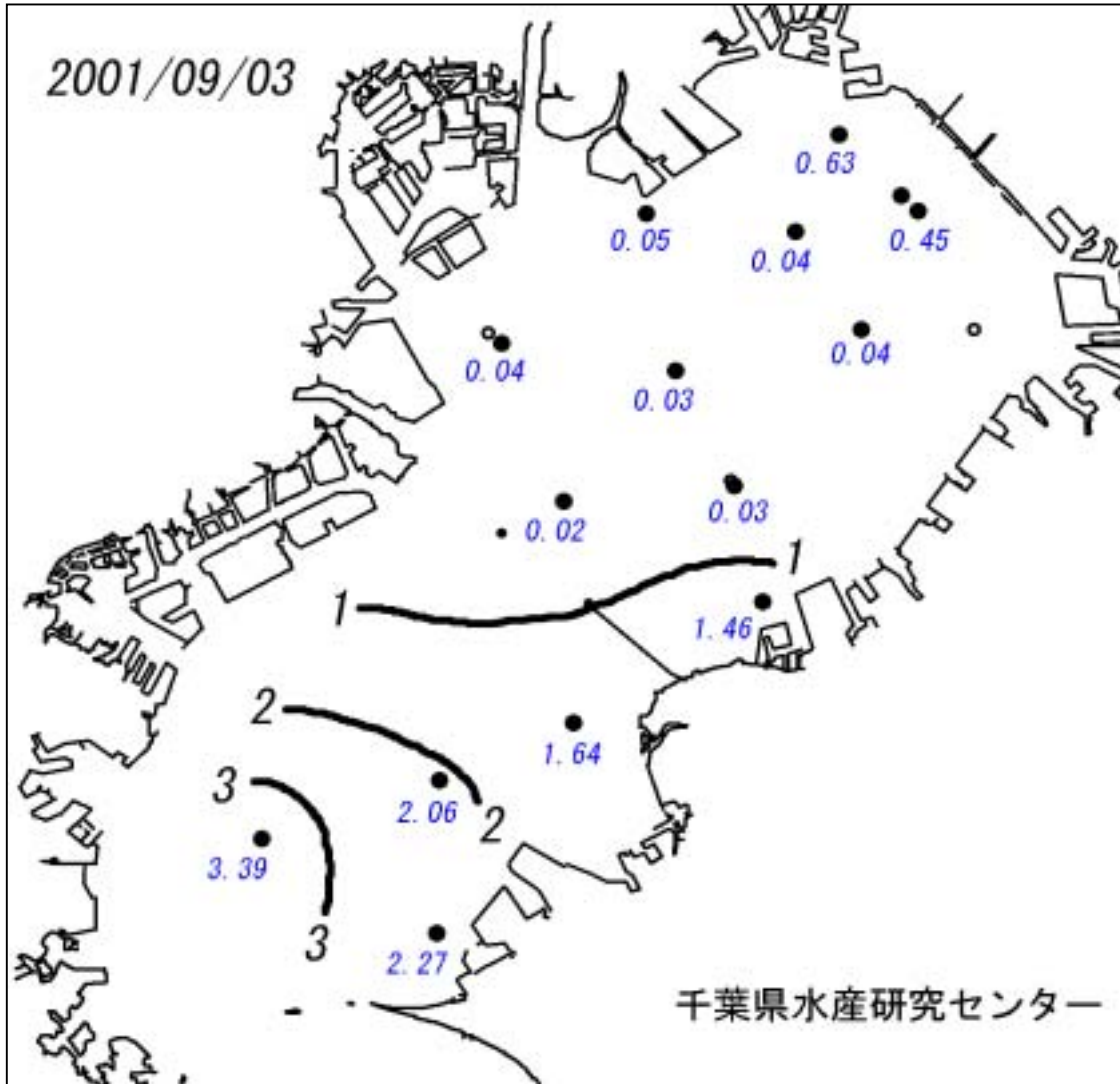
図 底層の溶存酸素量分布 (ml / L : 速報値) 平成13年9月3日観測分
