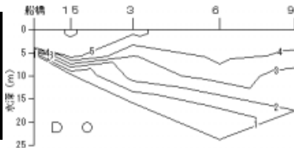
図 底層の溶存酸素量分布 (ml / L : 速報値) 平成13年9月3日観測分
