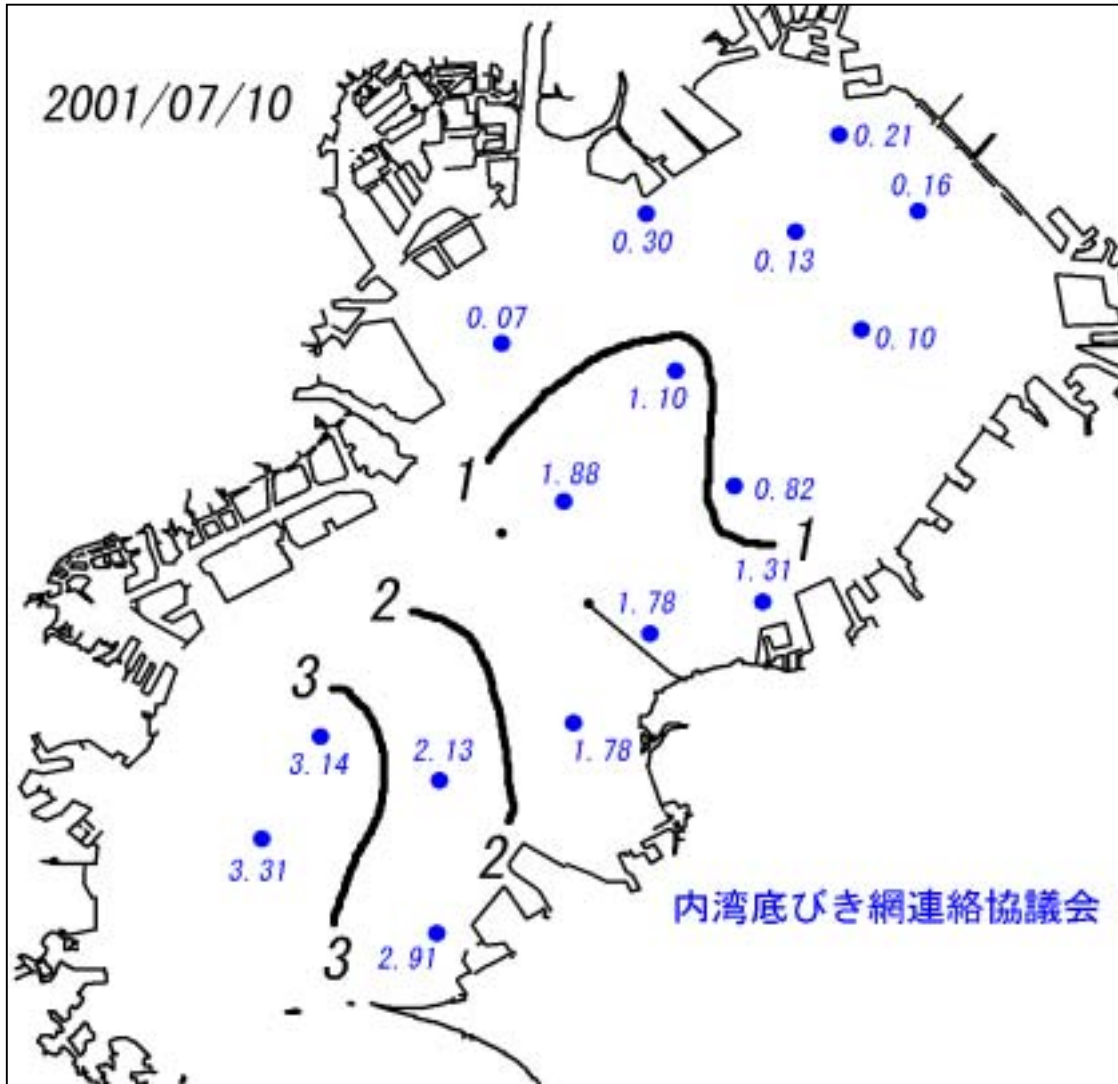
図 底層の溶存酸素量分布 (ml / L : 速報値) 平成13年7月10日観測分
