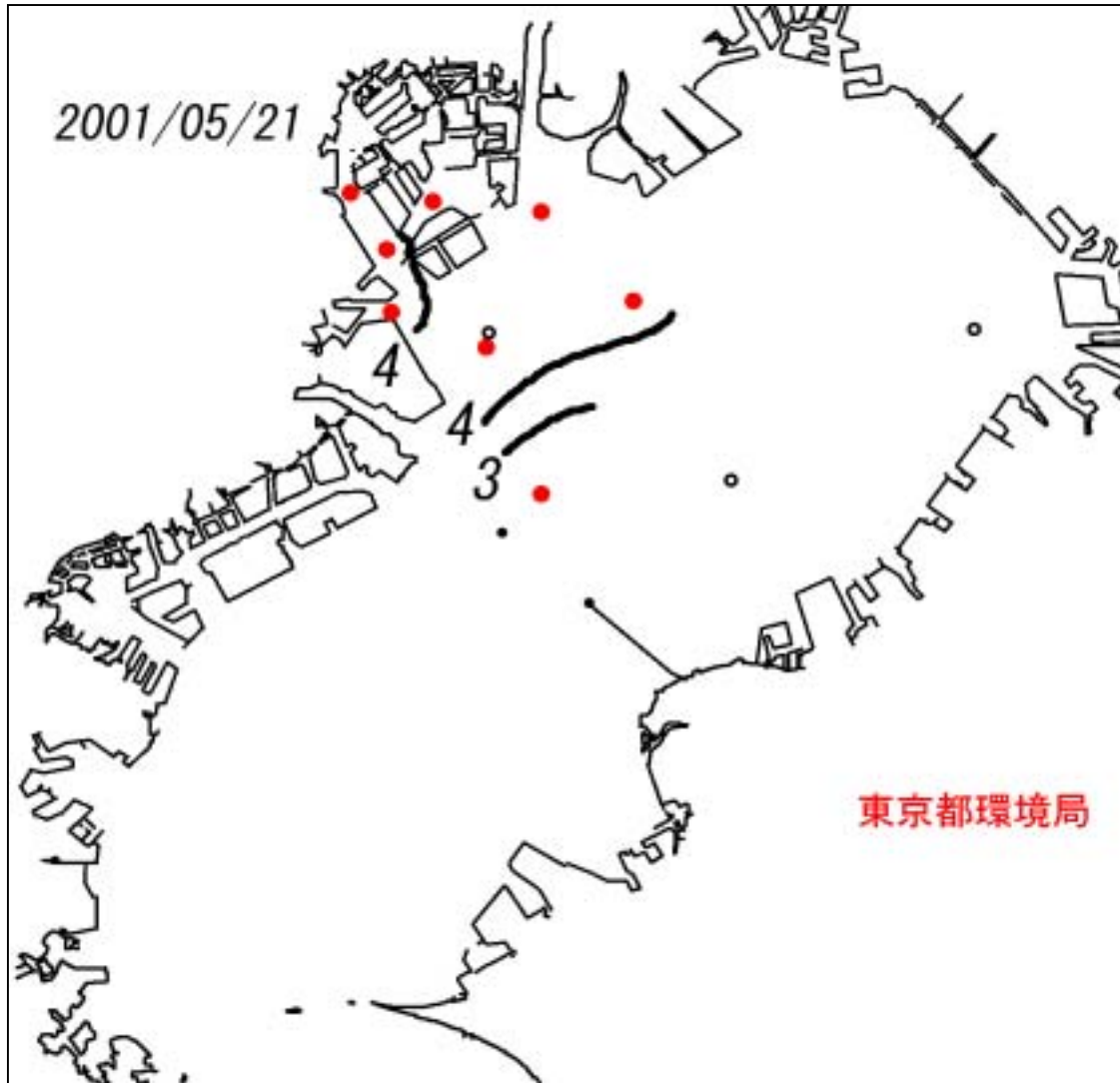
図 底層の溶存酸素量分布 (ml / L : 速報値) 平成13年5月21日観測分
