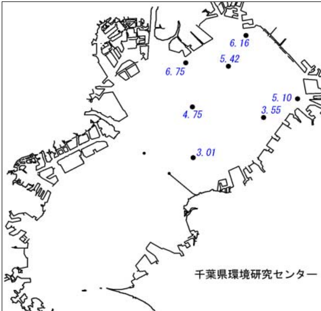
図 底層の溶存酸素量分布 (ml/L:速報値) 平成13年5月10日観測分
