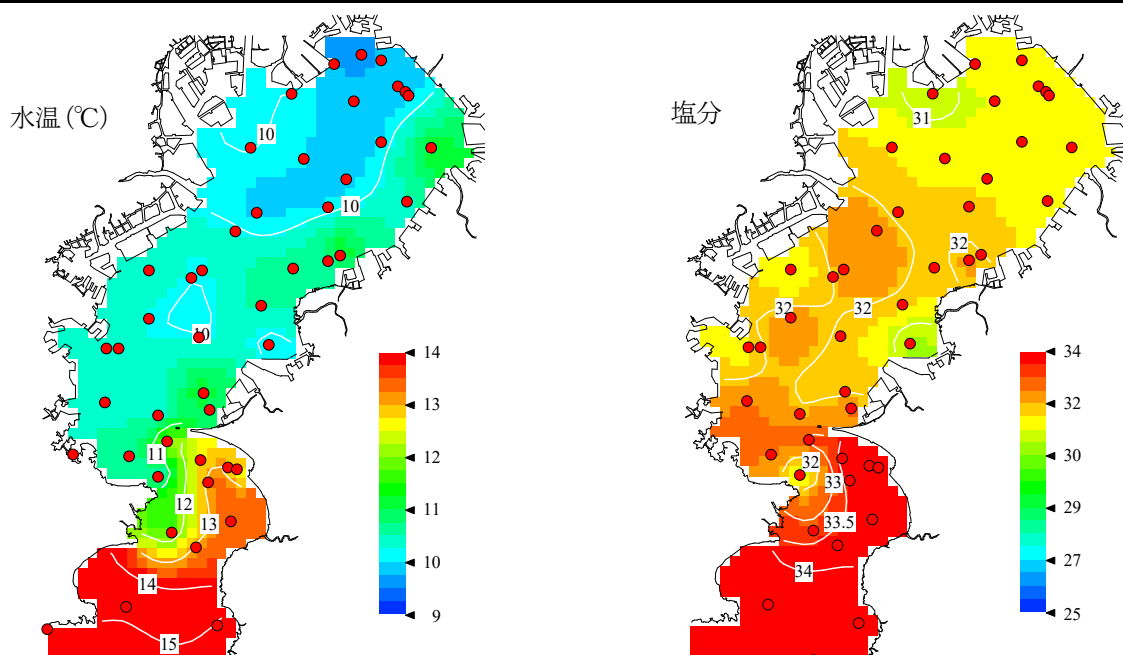
図1 表層の水温・塩分(平成31年3月1日)
