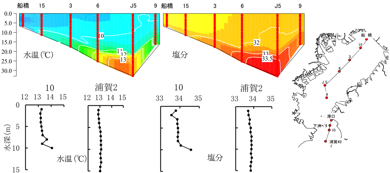
図2 縦断面の水温・塩分の鉛直分布(平成31年3月1日) 上：内湾(縦断面)、下：内房北部(グラフ)、右：調査ライン
