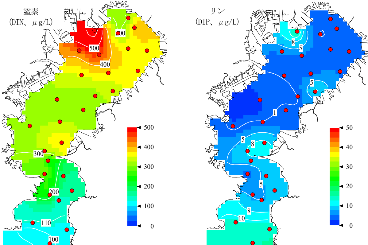
図 3 表層の栄養塩濃度の分布(平成 31 年 3 月 1 日)
