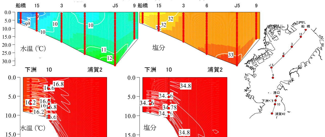
図2 縦断面の水温・塩分
